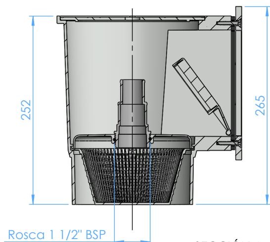
SECCIÓN A-A
