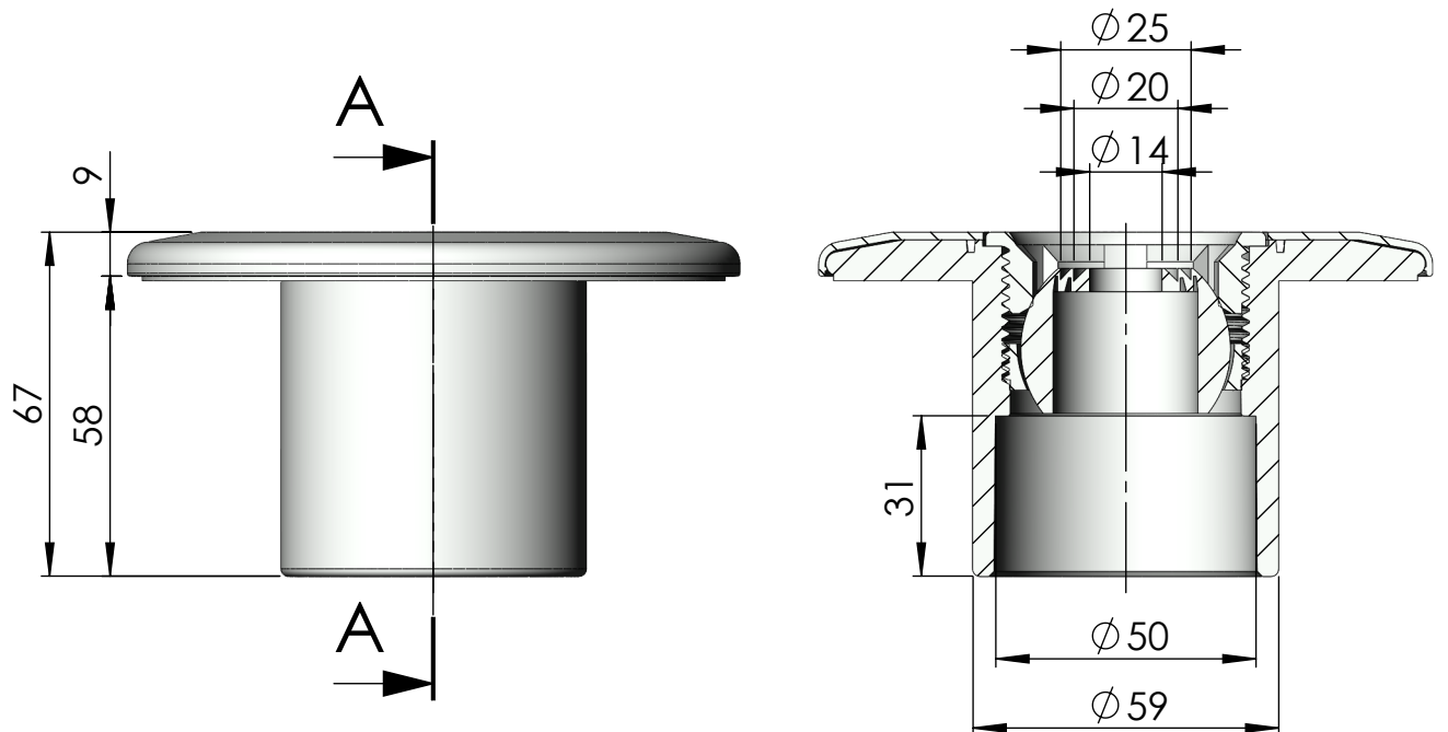
SECCIÓN A-A
