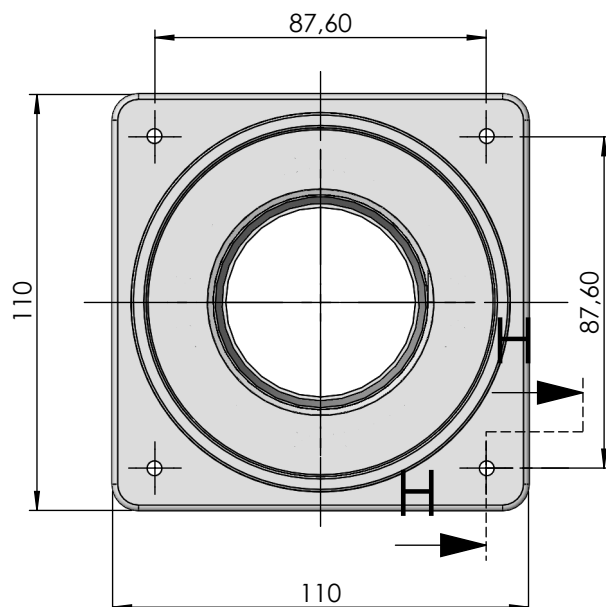
SECCIÓN H-H
