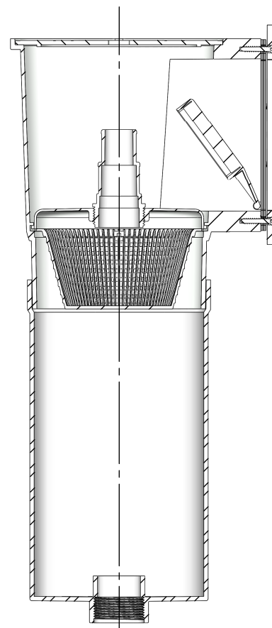
SECCIÓN A-A
