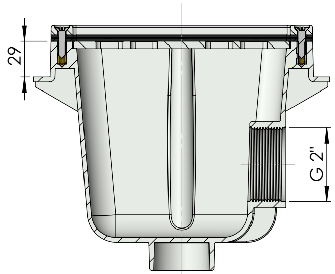
SECCIÓN B-B
