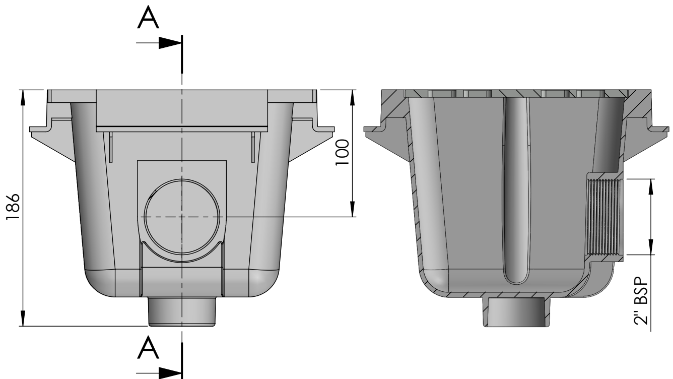
SECCIÓN A-A
