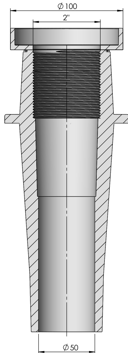
SECCIÓN A-A
