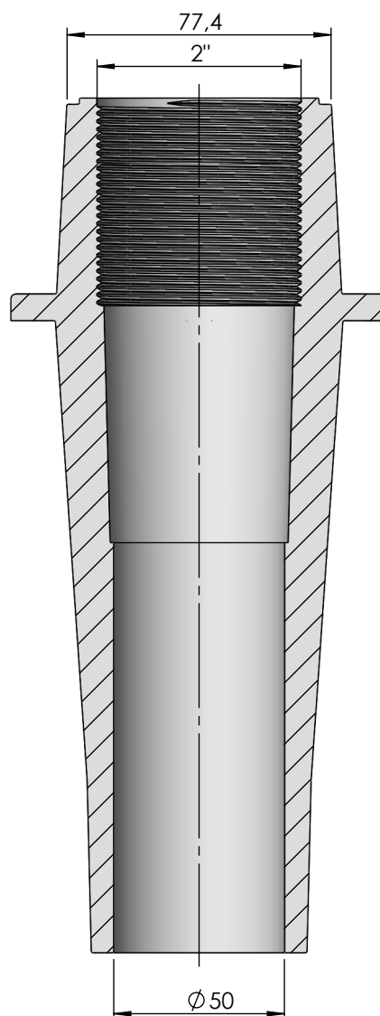
SECCIÓN A-A
