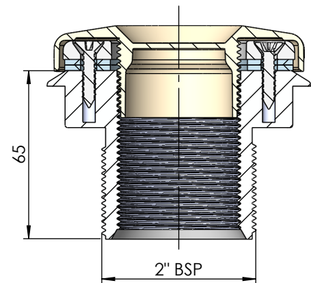
SECCIÓN A-A
