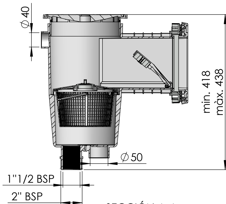
SECCIÓN A-A
