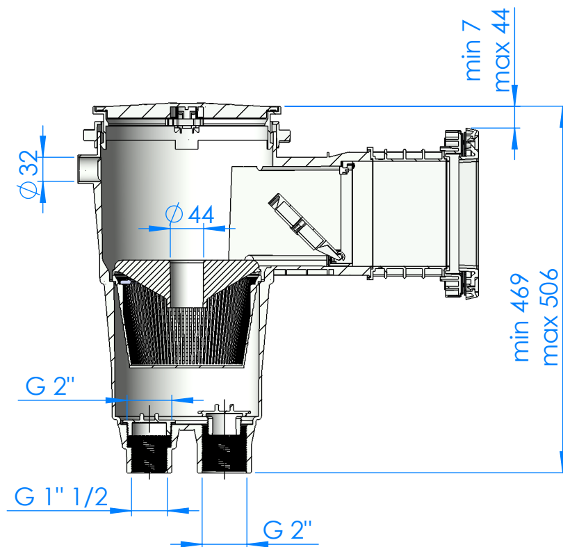
SECCIÓN A-A
