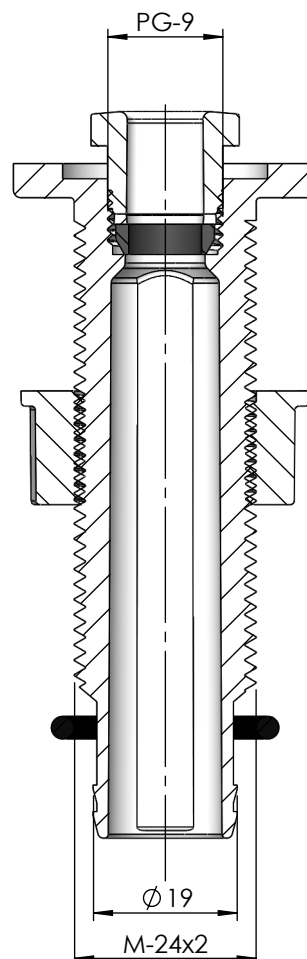
SECCIÓN A-A
